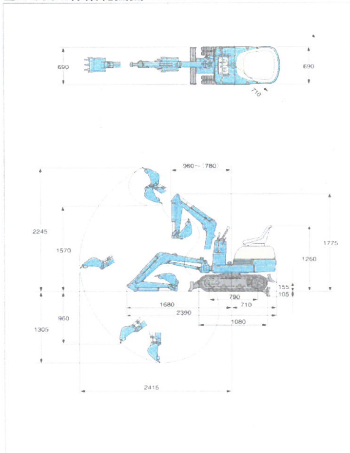
■K-005-3作業範囲図 単位:mm
