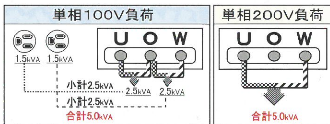
※発電出力は合計で5.0kVA (単相3線出力端子:1組、単相100Vコンセント:15A×2個)
